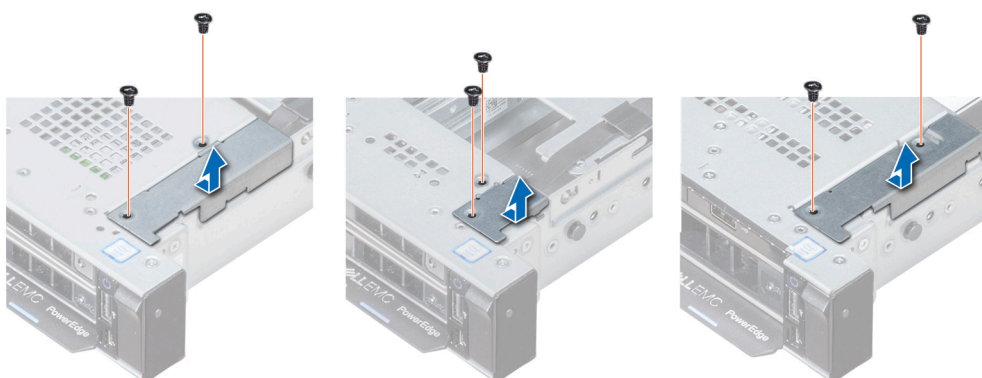
Ilustración 123. Extracción de la cubierta de cables
