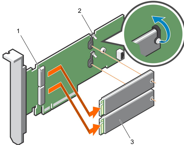
Ilustración 67. Extracción del módulo M.2 SSD
